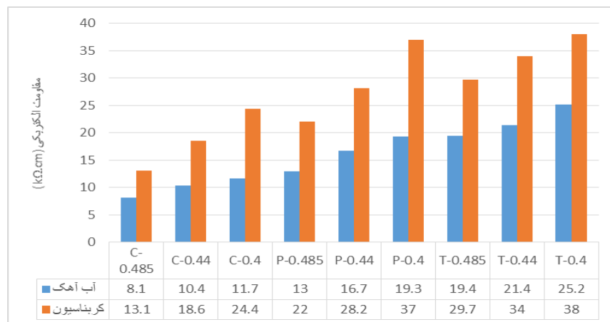
شکل ۸- مقایسه مقاومت الکتریکی ۱۱۹ روزه ملات‌های نگهداری شده در آب آهک و محیط کربن‌دی‌اکسید
