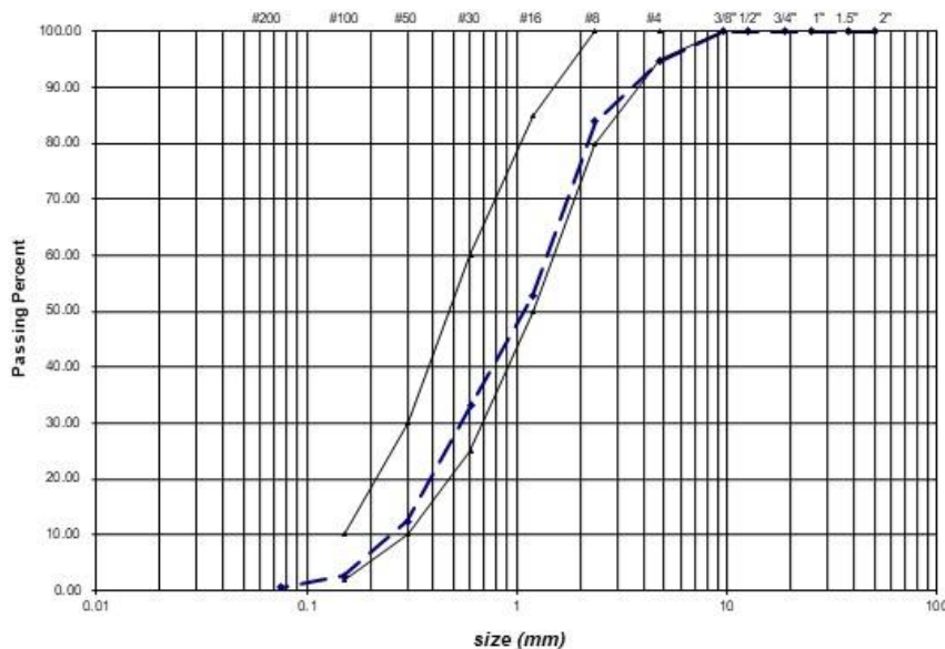
شکل ۱- نمودار دانه‌بندی ماسه مصرفی
