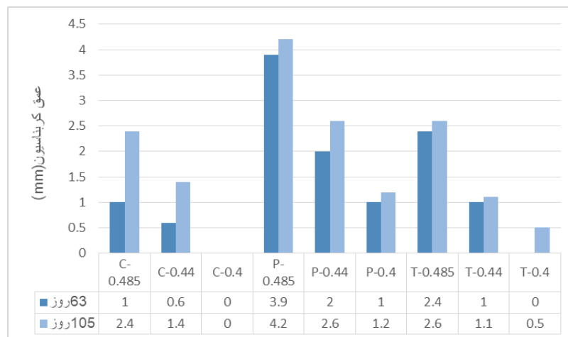
شکل ۳- عمق کربناسیون ملات‌ها پس از ۶۳ و ۱۰۵ روز مجاورت با گاز کربن‌دی‌اکسید
